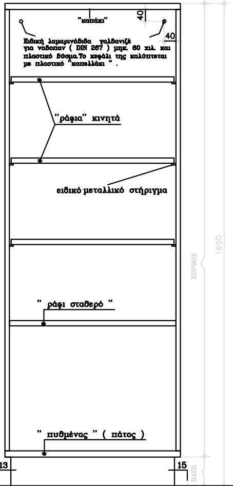
ΟΨΗ ΧΩΡΙΣ ΤΑ ΝΤΟΥΛΑΠΟΦΥΛΛΑ 1:10
