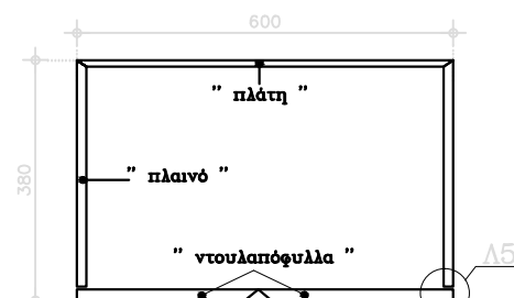
"ΚΟΡΜΟΣ" ΤΟΜΗ 1-11 1:10
