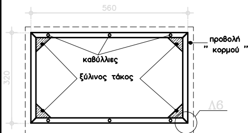
"ΒΑΣΗ" - ΤΟΜΗ 13-15 1:10
