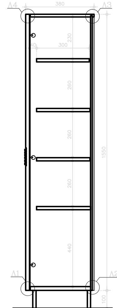
ΤΟΜΗ 2-10 1:10
