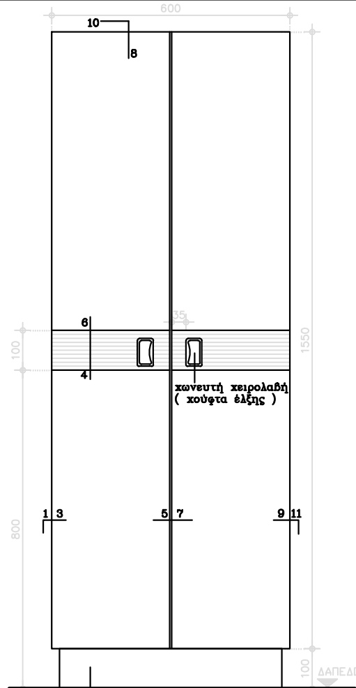
ΟΨΗ 1:10
